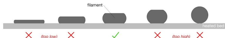
Bild 10 - So stimmen Sie die Düsenhöhe während des Testdrucks live ab. Hinweis: -0,640 mm dient nur zur Veranschaulichung. Ihre Einstellung wird verschieden sein!
