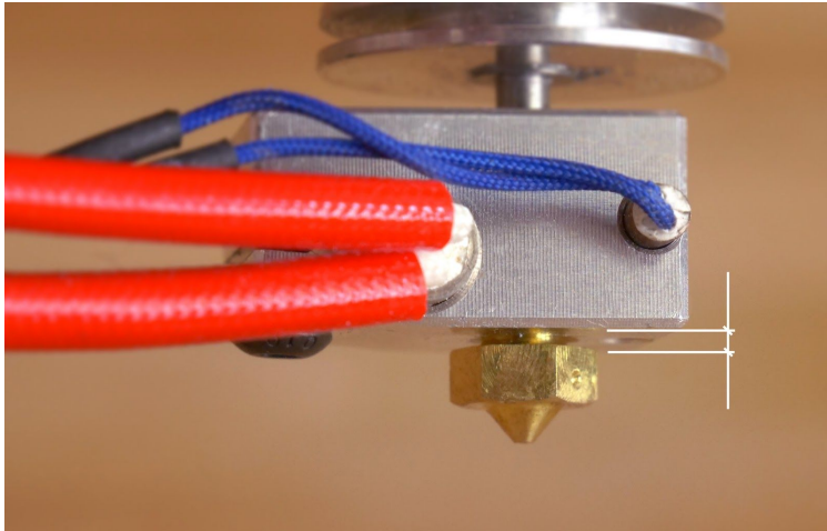
Bild 41 - Ein Spalt zwischen einer vollständig eingeschraubten Düse und dem Heizblock
