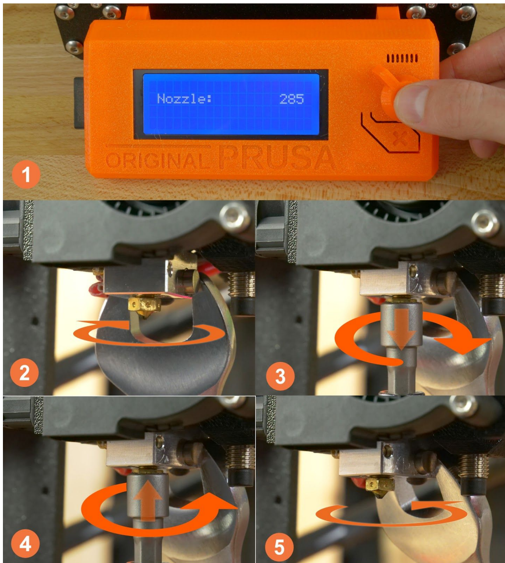
Bild 42 - Düsenwechsel
