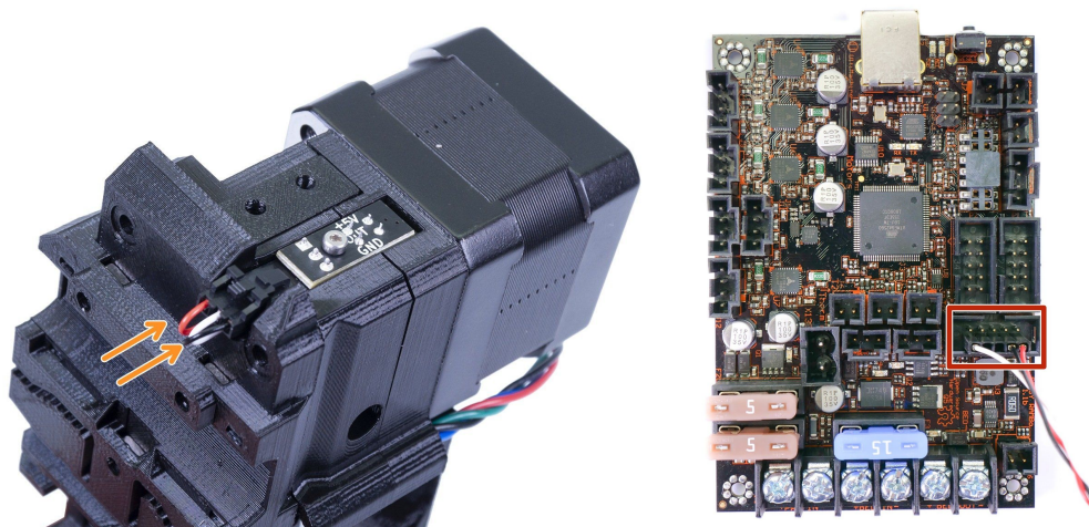
Bild 38 - Korrekt angeschlossener und sitzender Filamentsensor
