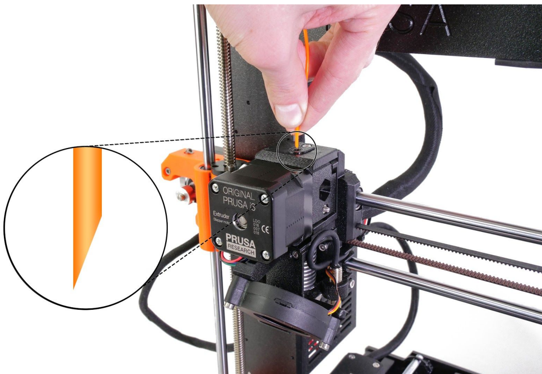
Bild 9 - Einlegen des Filaments in den Extruder
