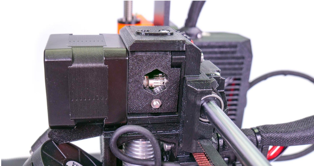
Bild 40 - Reinigen des Extruders - hier sehen Sie die Antriebsritzel durch das Wartungsloch
