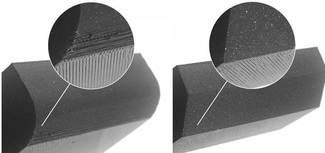
Bild 28 - Verrundung (links) vs. Fase (rechts)
