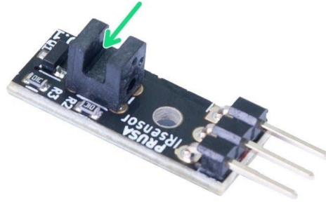
Bild 39 - IR-Filamentsensor
