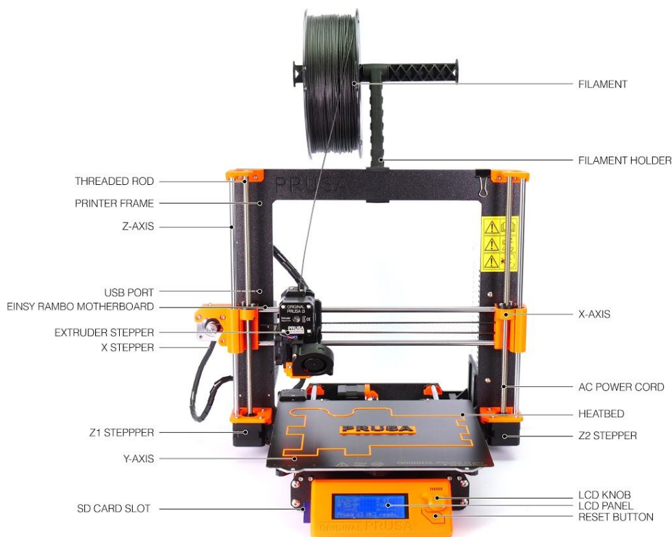
Bild 1 - Original Prusa i3 MK3S Drucker Beschreibung
